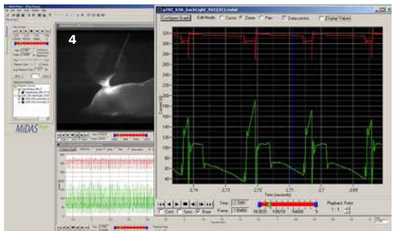
Echtzeitlaboraufnahmen zeigen den kontrollierten IACT Prozess auch während der Schweißtropfenablösung.
